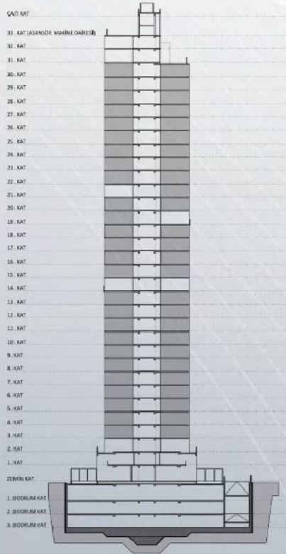
B BLOK KESİTİ
