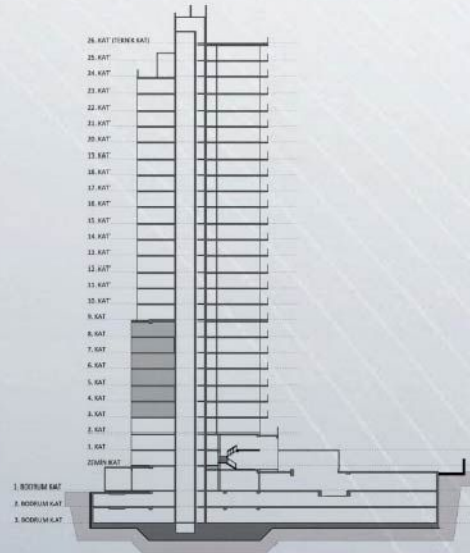
A BLOK KESİTİ
